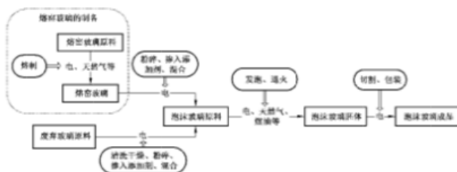
图1 泡沫玻璃生产企业能源消耗统计流程图
