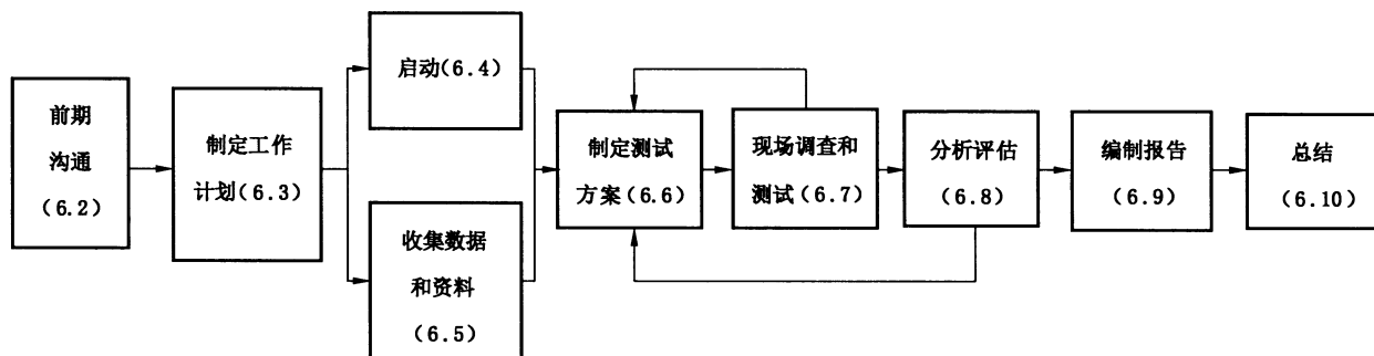
图1 能源审计流程图
